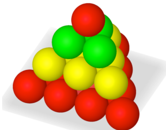
Empilement A-B-C-A de 20 sphères
