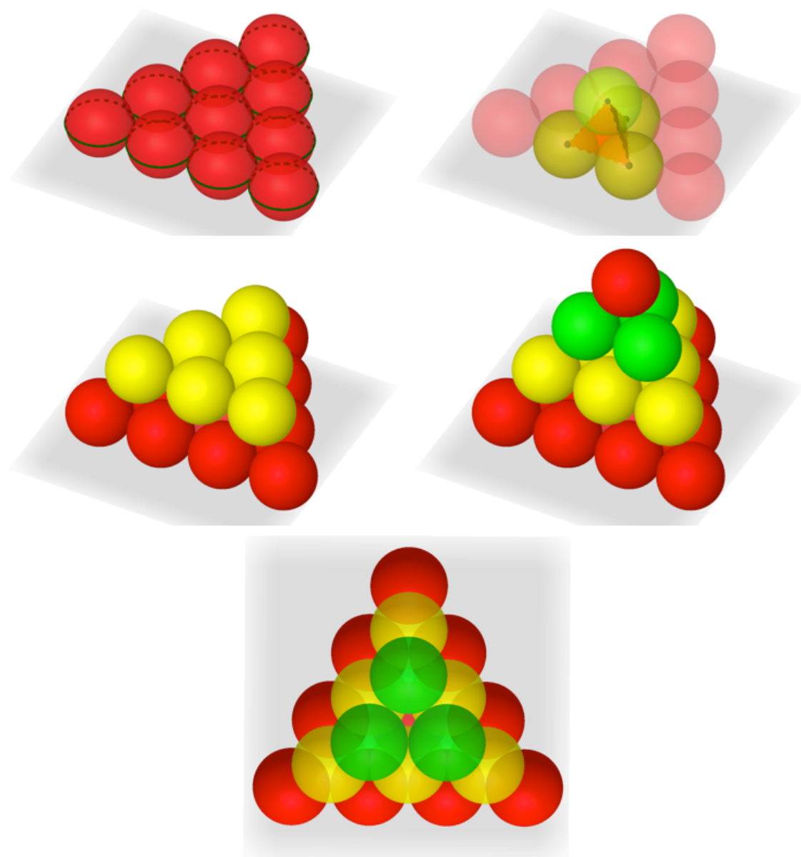
Empilement A-B-C vu du dessus
