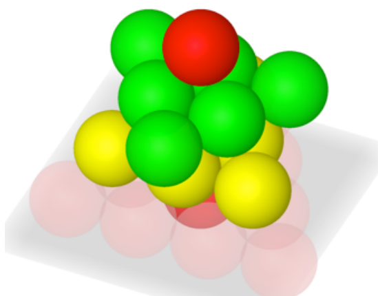
Ne garder que la sphère centrale la 1 re couche A pour faire apparaître les sphères aux sommets d'un cube et au centre de ses faces.
