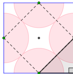
Vue du plan médian de face
